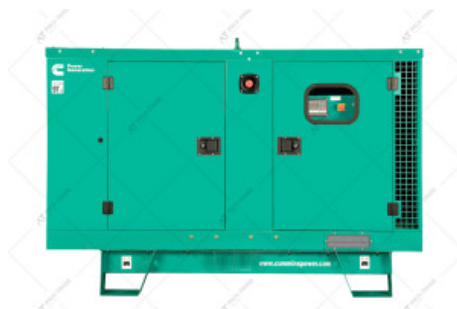
№10371 Дизельний генератор Cummins C22D5Q 18/16 кВт відкритого типу
